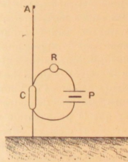
Fig. 7. — Appareil récepteur.
