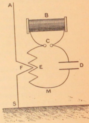
Fig. 8. — Transmetteur Marconi.
