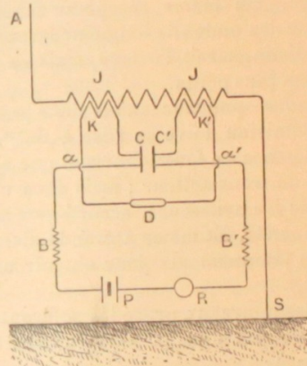
Fig. 9. — Récepteur Marconi.
